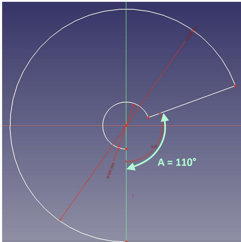
Cotes du gabarit
